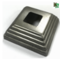
Основание балясины, арт. R10436.02 80х80х1мм, кв.25х25мм Вес: 0.075 кг Цена (за шт): 10 руб.
